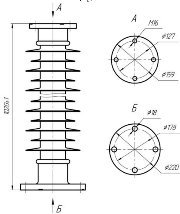
Технічні характеристики фактично витриманих величин ізолятора
