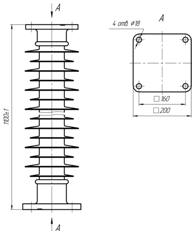
Технічні характеристики фактично витриманих величин ізолятора
