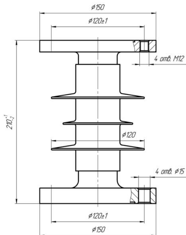
Технічні характеристики фактично витриманих величин ізолятора
